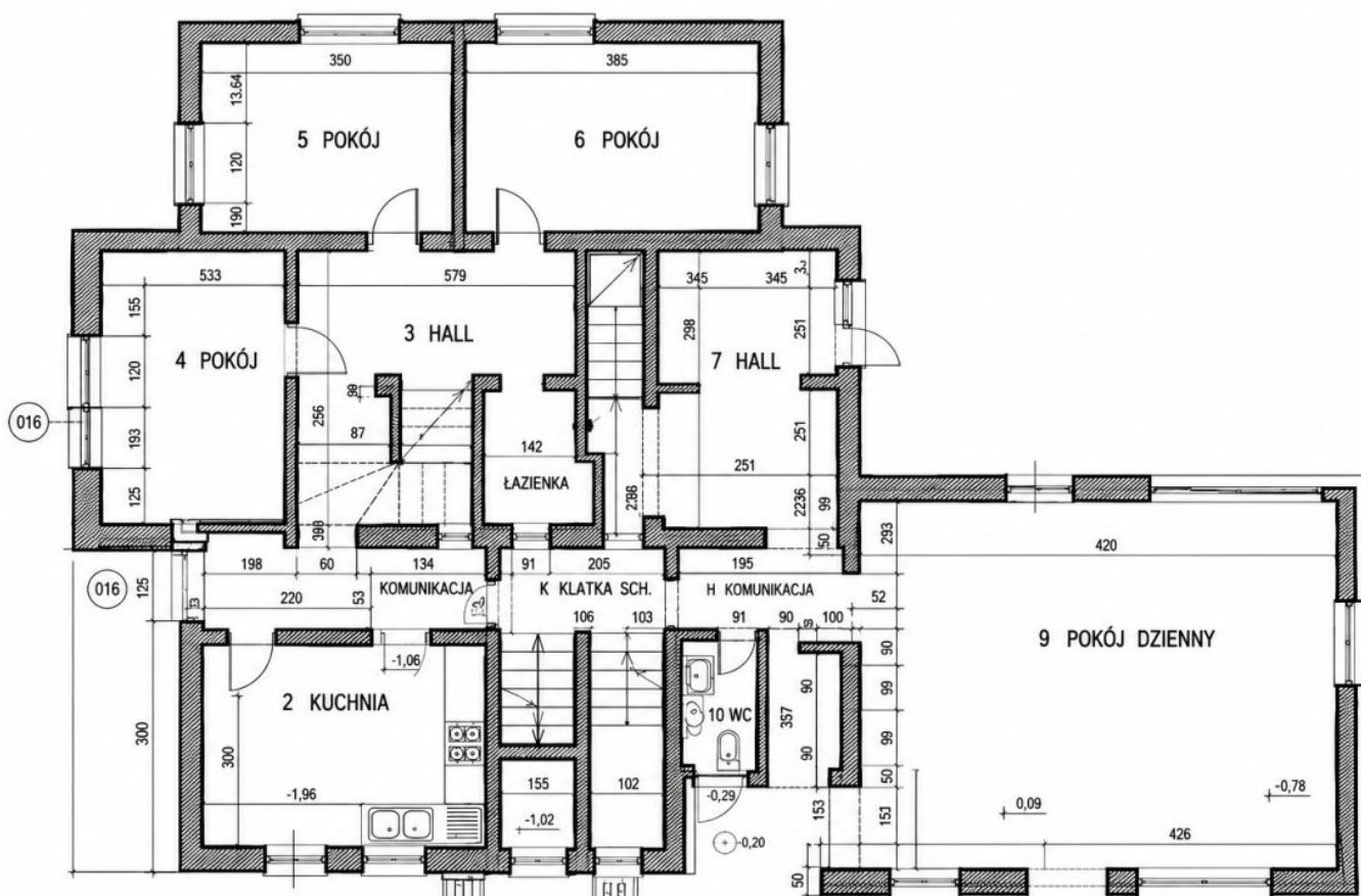
RZUT PARTERU 1:1
