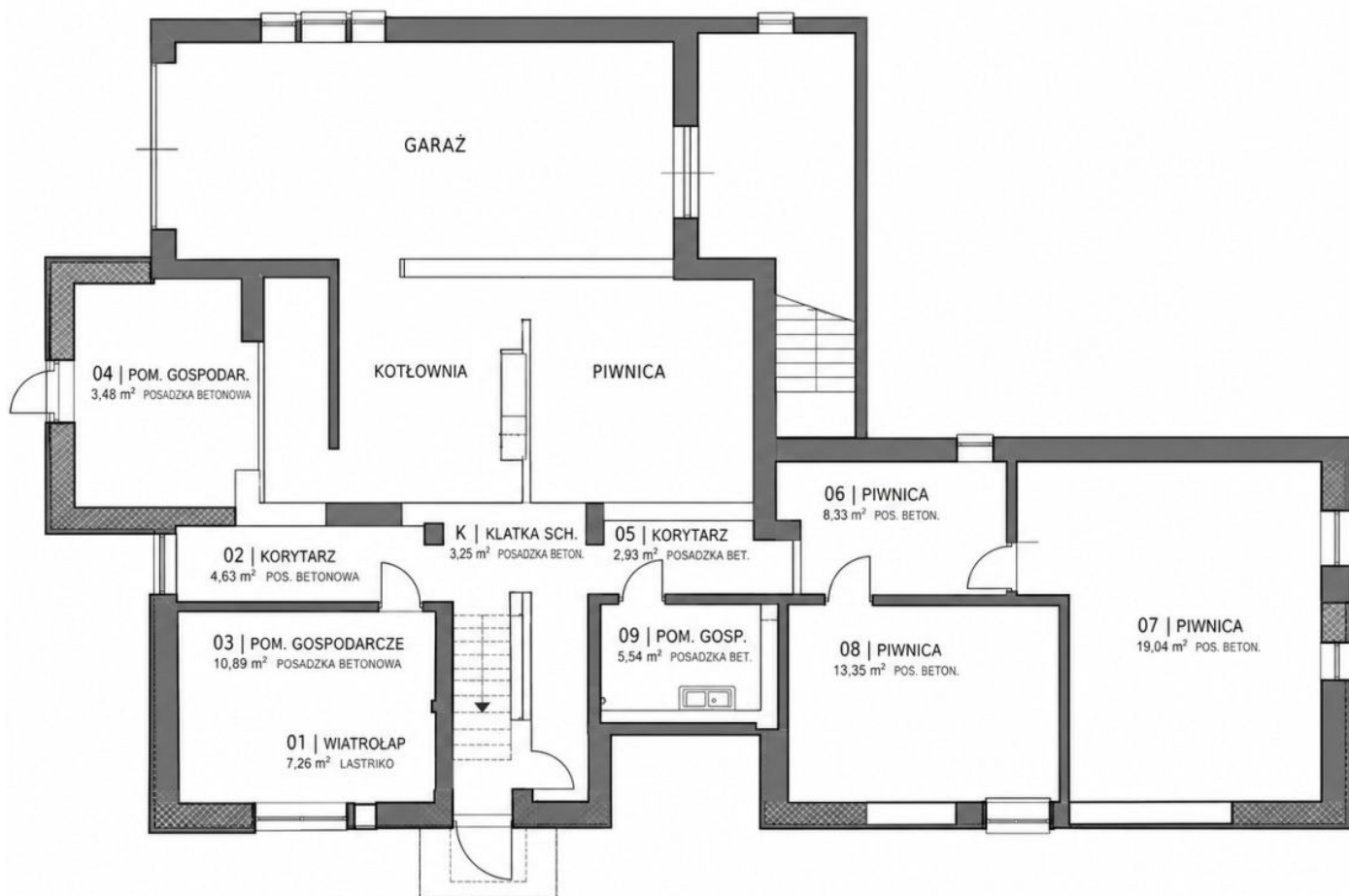
RZUT PIWNIC 1:50
