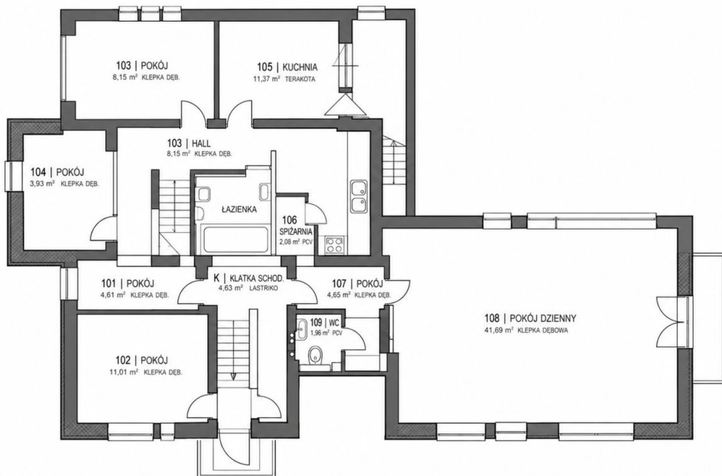
RZUT PIĘTRA 1:50
