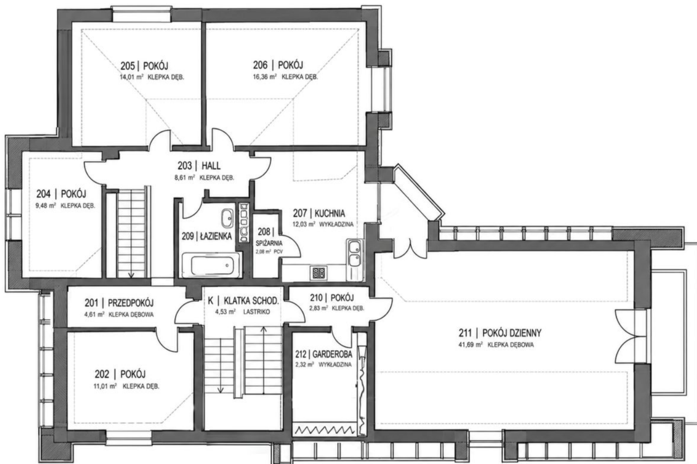
RZUT PODDASZA 1:50
